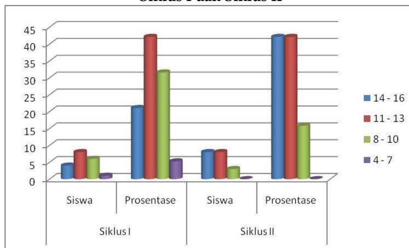
Gambar 4.7 Grafik Batang Perbandingan Keaktifan Belajar dan Tes Kemampuan Menghafal Siklus I dan Siklus II
